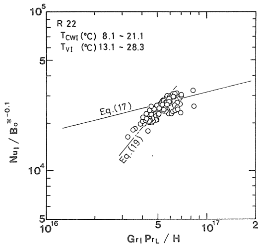
Fig. 10 Nu_t / Bo^{*-0.1} \sim Gr_t Pr_L / H
