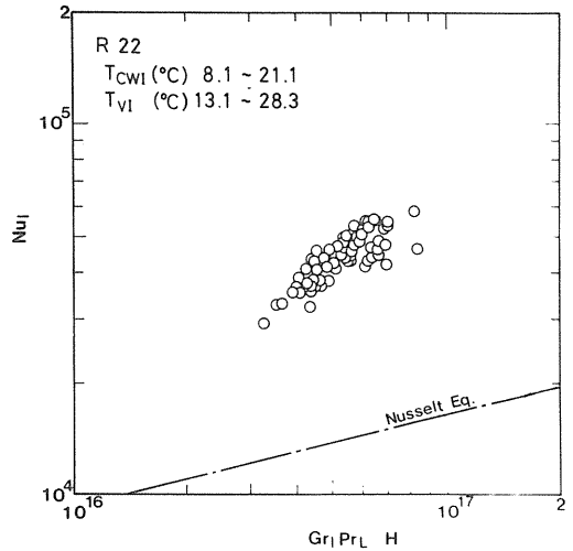
Fig. 8 Nu_i versus Gr_i Pr_L / H
