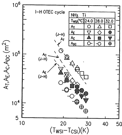
図10 伝熱面積
