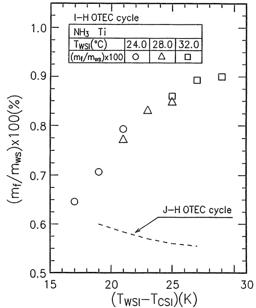
図9 淡水化比
