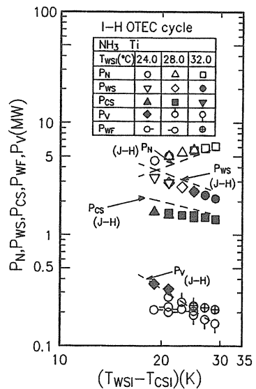
図6 正味出力とポンプ動力
